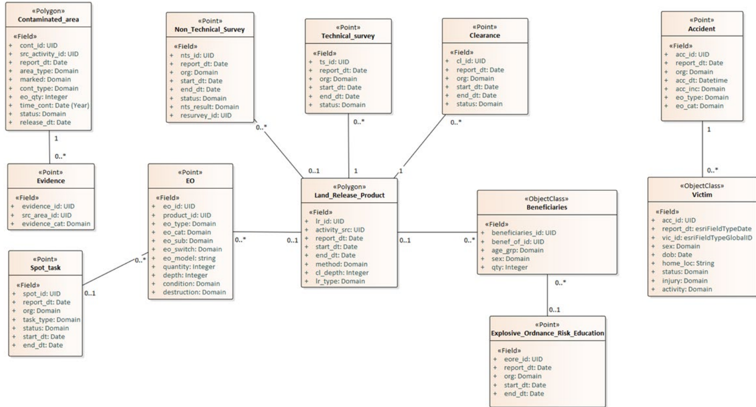
الشكل ب.1 – هيكل البيانات
